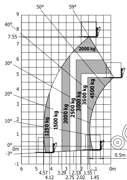
Abaque tout-terrain (EN 1459 B)
