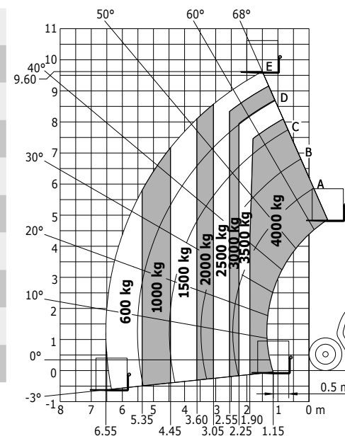
Abaque tout-terrain (EN 1459 B)
