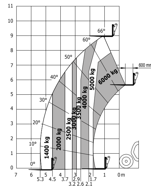
Abaque industriel (EN 1459 A)
